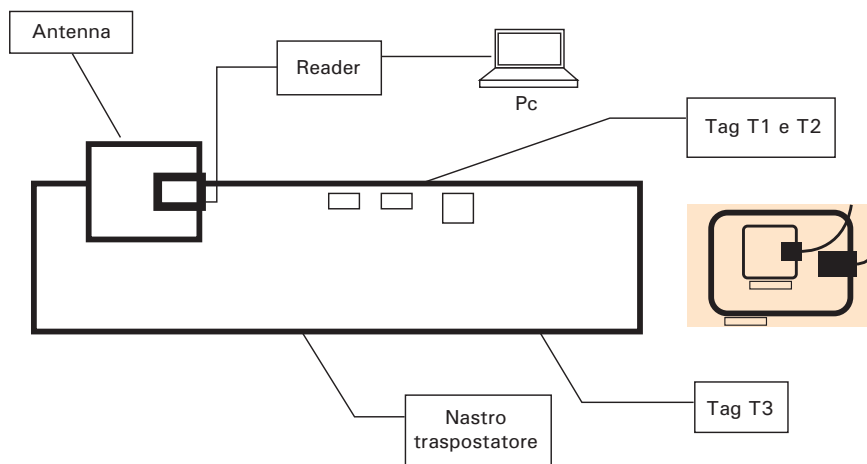
Schema del sistema utilizzato per le prove.
