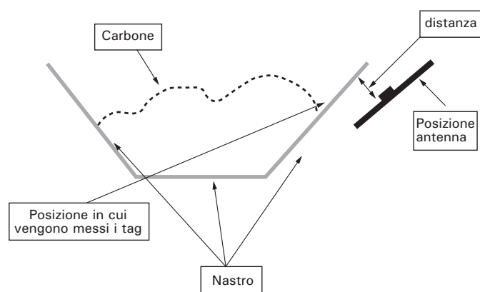
Schema di posizionamento dell'antenna.
